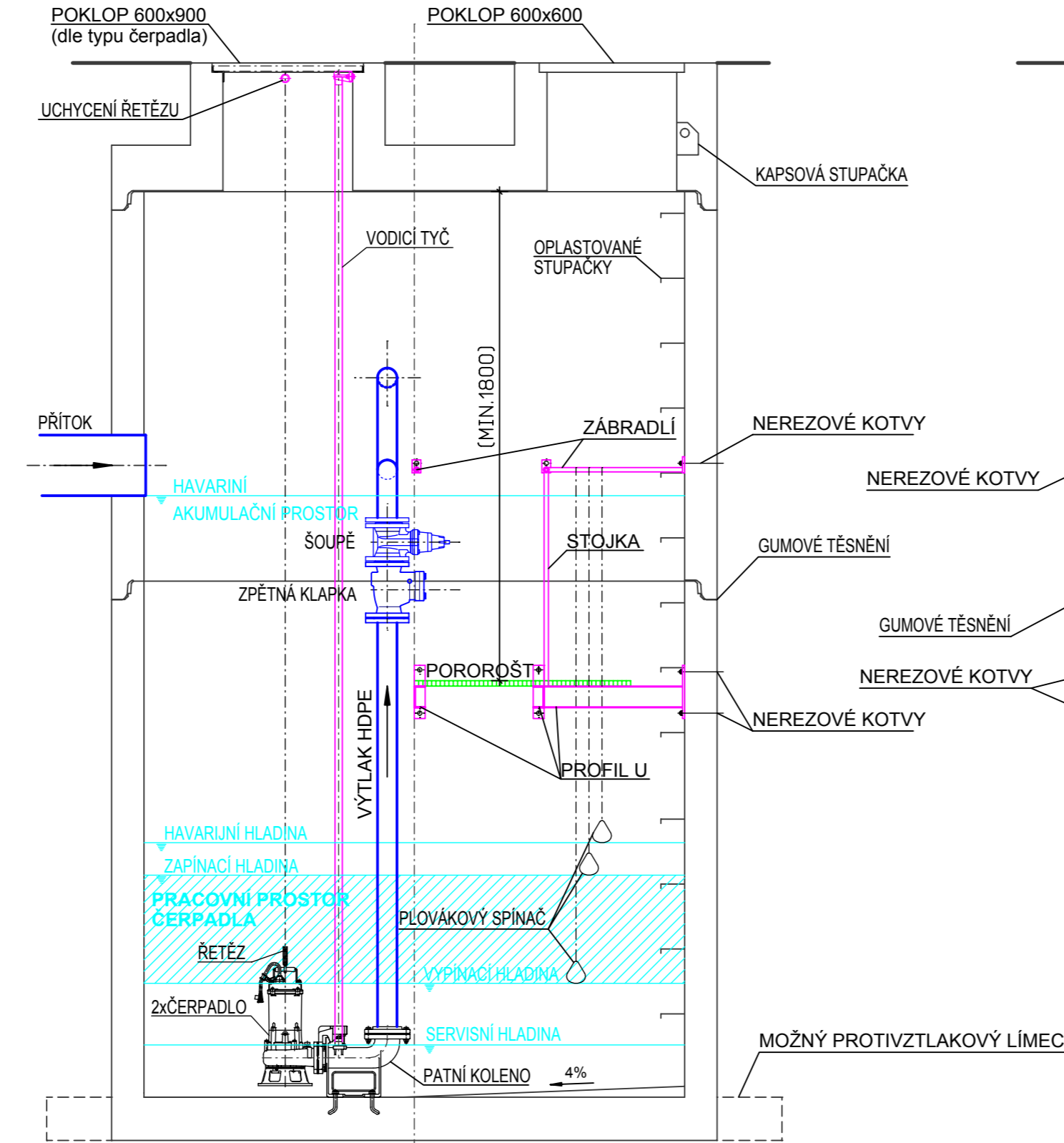
ŘEZ A-A
