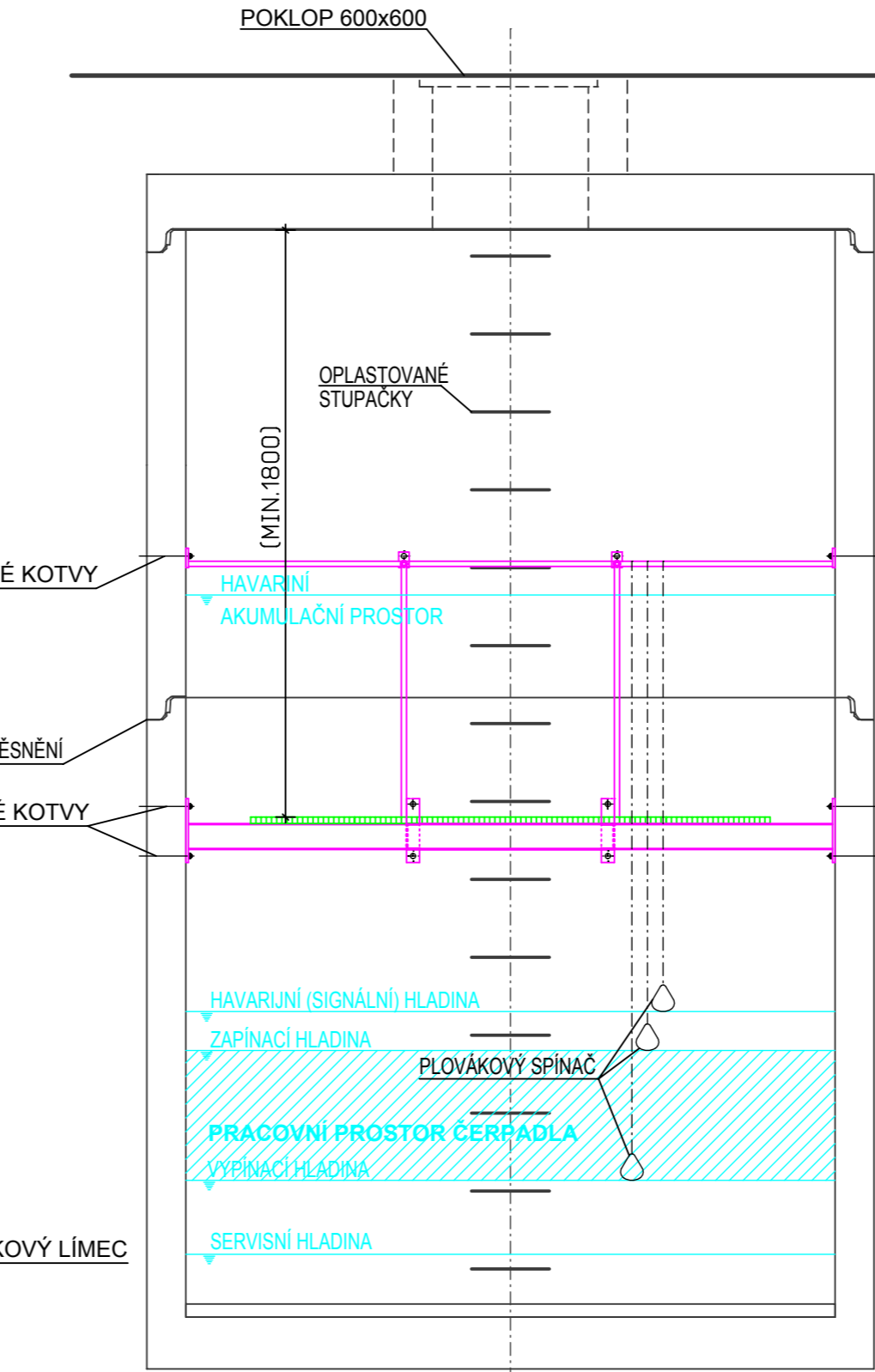
ŘEZ C-C
