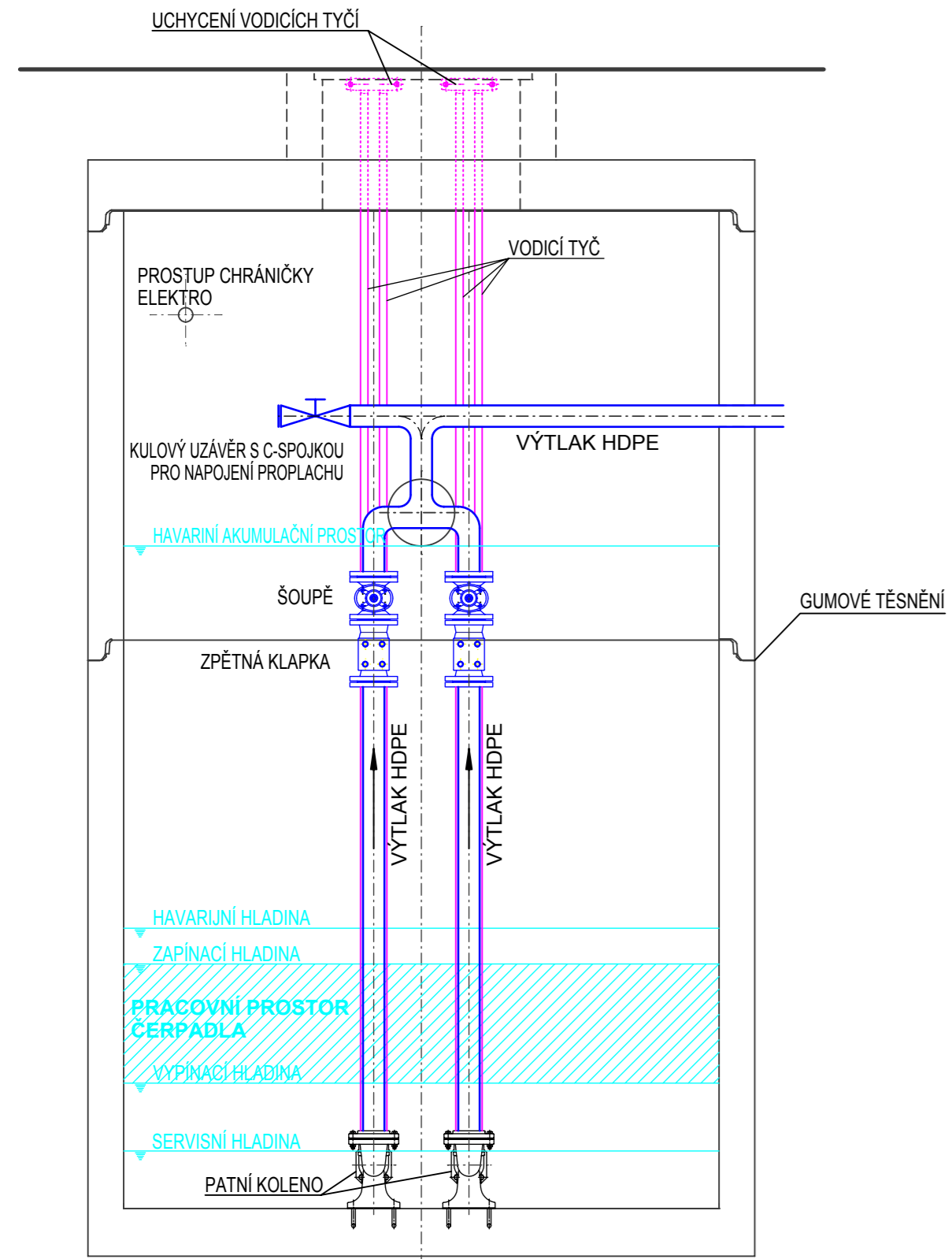
ŘEZ B-B
