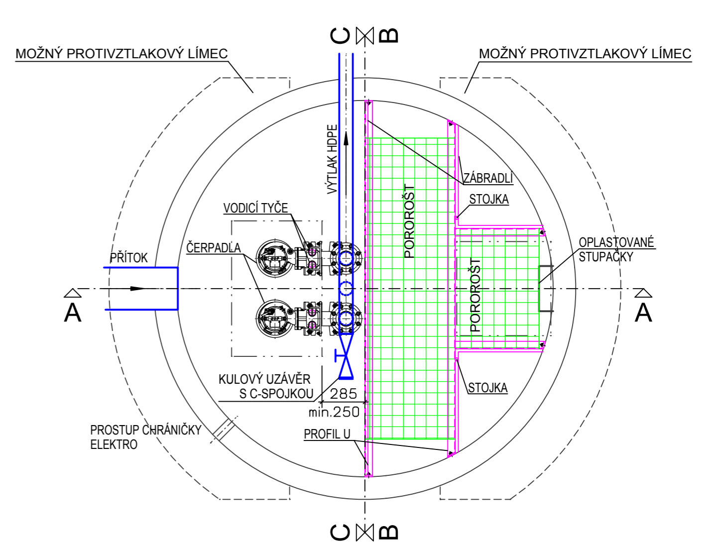
PŮDORYS
