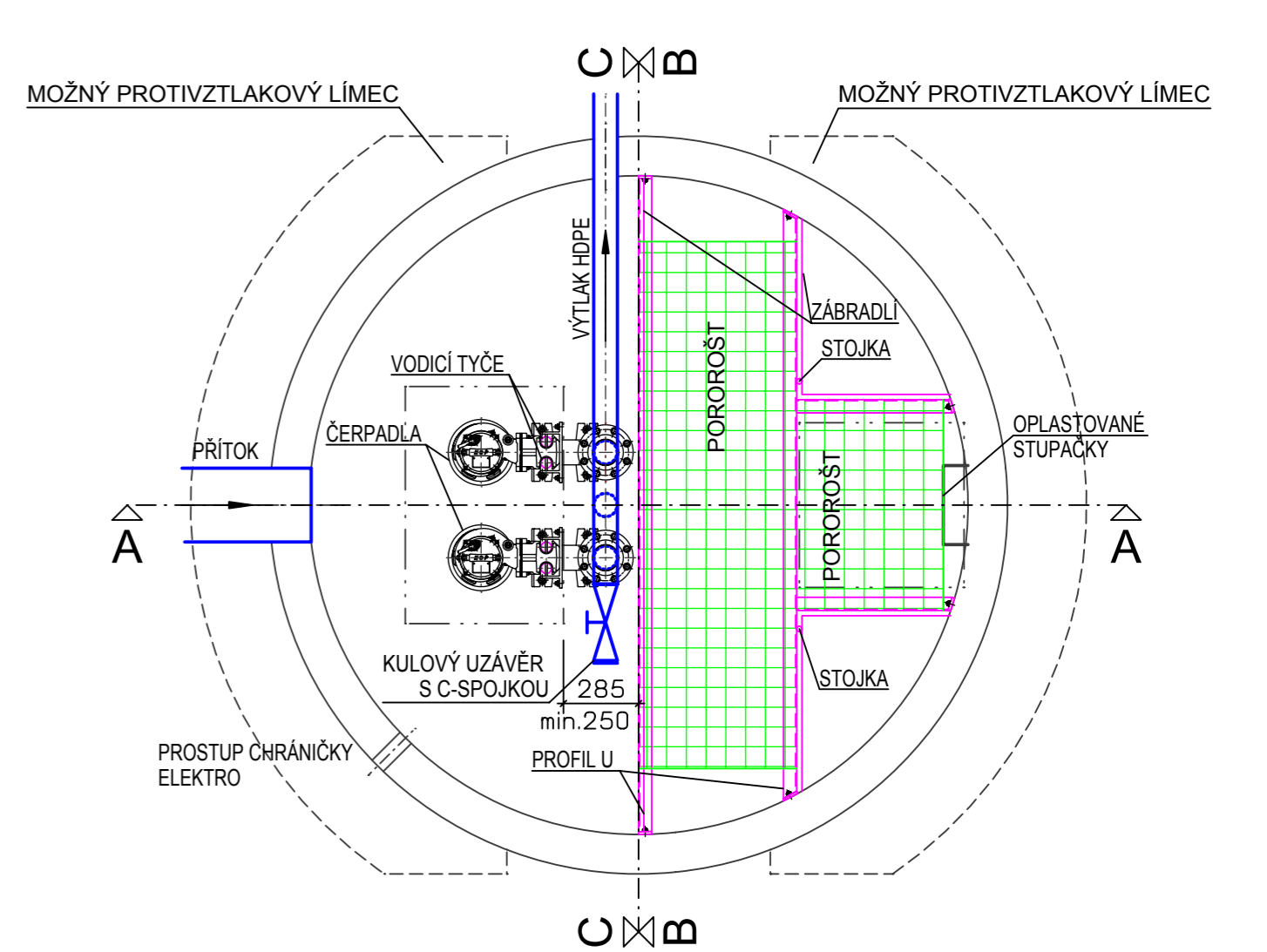
PŮDORYS
