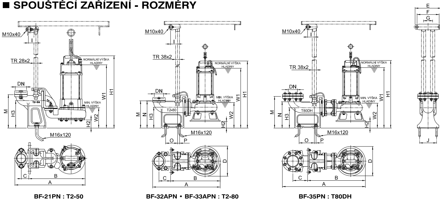
BF-21PN : T2-50
