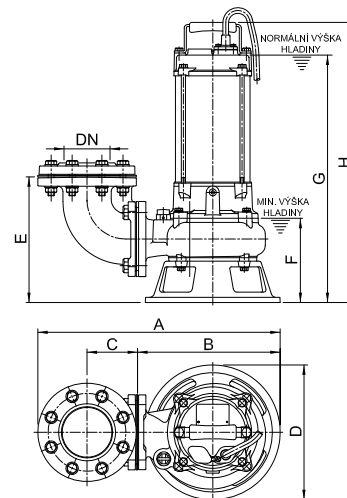
BF-35PN
